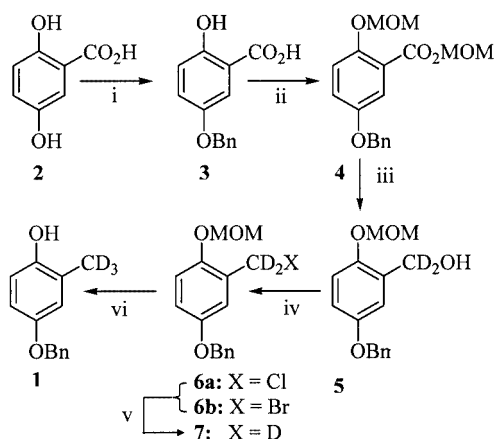
Scheme 1. i) NaH, DMF then BnBr, 86%; ii) NaH, DMF then MOMCl, quant.; iii) LiAlD 4 , THF, 86%; iv) MeSO 2 Cl, 2,6-lutidine, excess LiBr, THF, 85%; v) LiAlD 4 , THF, 90%; vi) MeOH, cat. p -TsOH, 50 °C, 3 h, 95%
